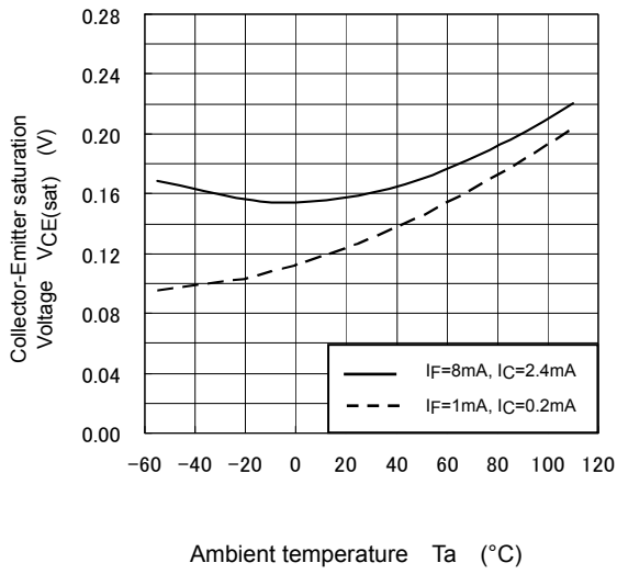
V_{CE(sat)} - T_a
