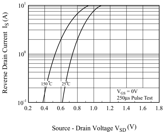
Fig5. I_S - V_{SD}
