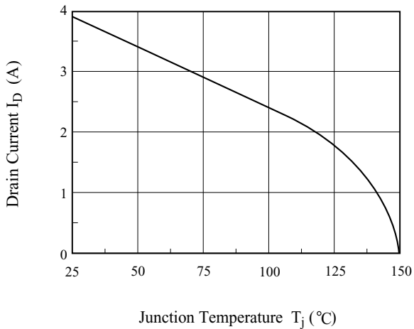
Fig11. I_D - T_j
