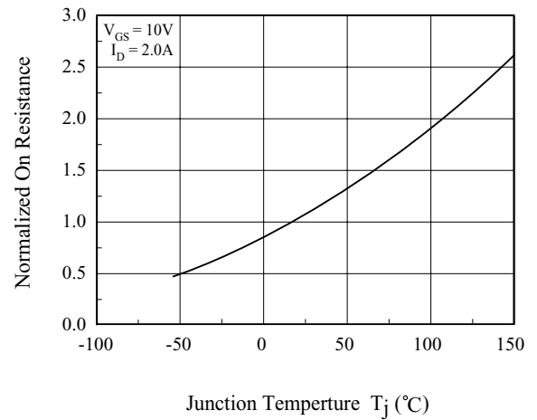
Fig6. R_{DS(ON)} - T_j
