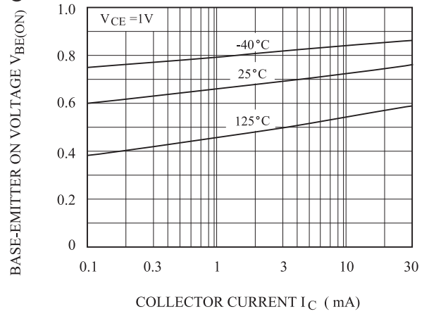
V_{BE(ON)} - I_C
