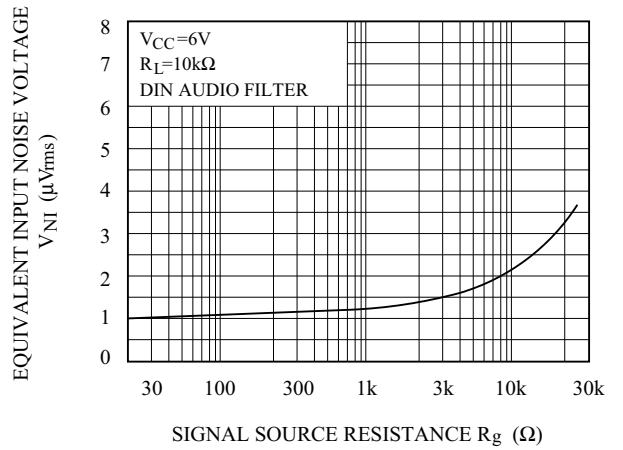
V_{NI} - R_g
