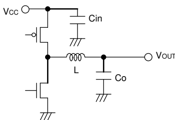
Fig.98 Input capacitor
