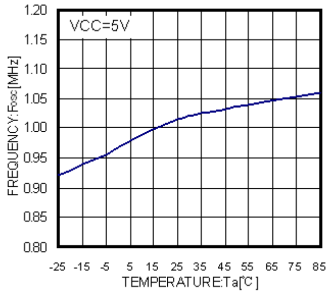
Fig.15 T_a - F_{osc}
