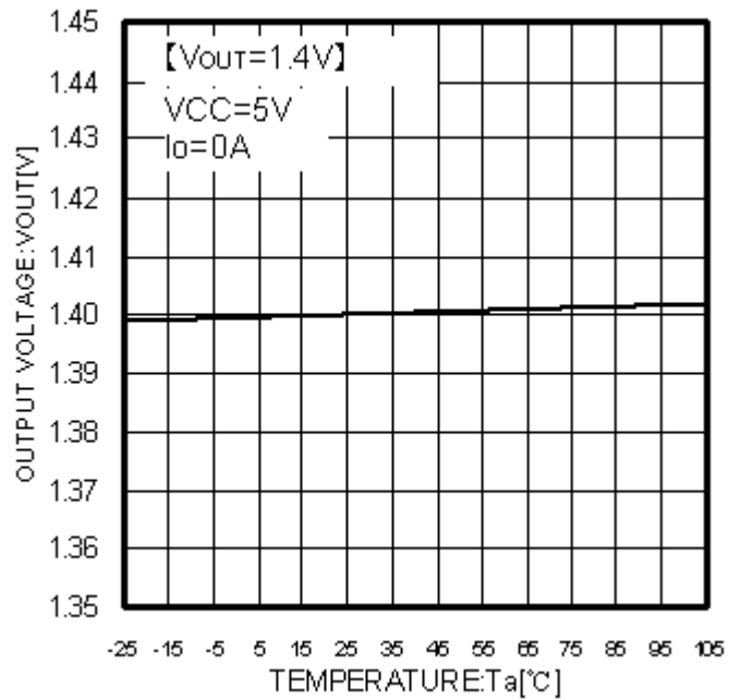
Fig. 58 Ta-Vout
