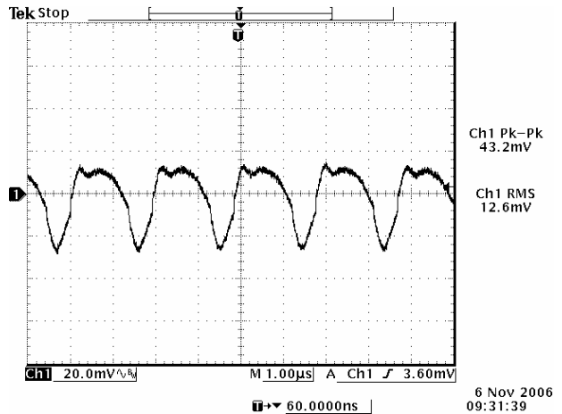
12 V input, 3.3 V output
