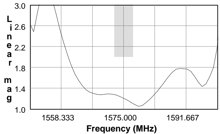
S11 VSWR
