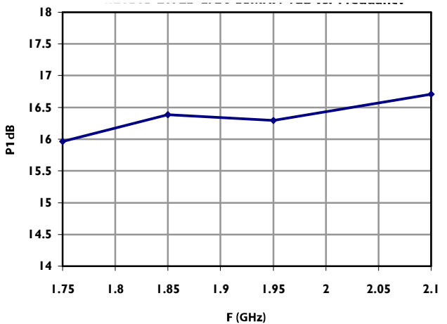
P1dB
