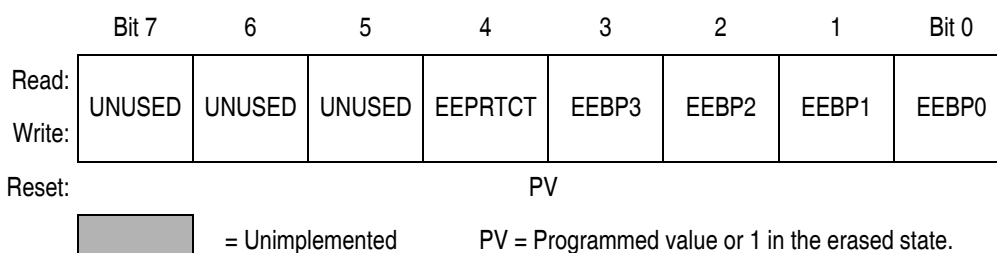
Figure 5-4. EEPROM-1 Nonvolatile Register (EE1NVR)
