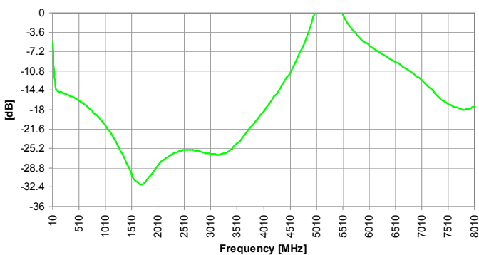
CMRR
