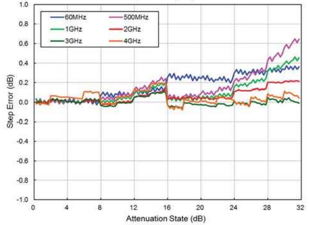
Step Error (dB)
