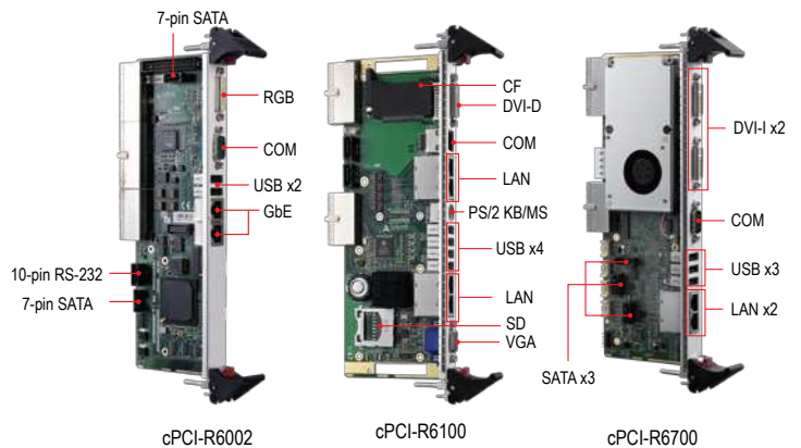
cPCI-R6002
