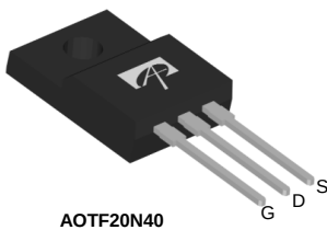
AOTF20N40
