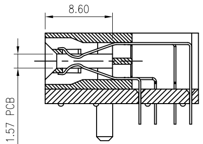
A-A SCALE 2:1
