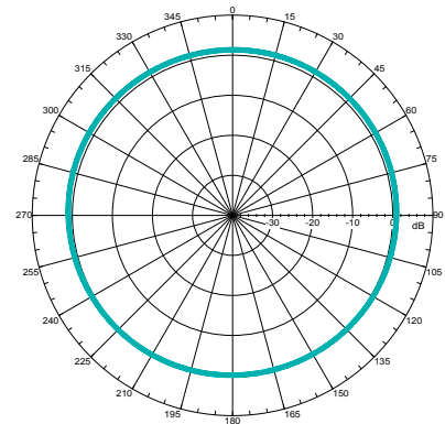
2.5GHz 1.38176dBi
