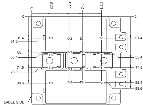
Tr1 / Tr2: IGBT, Di1 / Di2: FWDi
