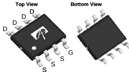
SOIC-8
