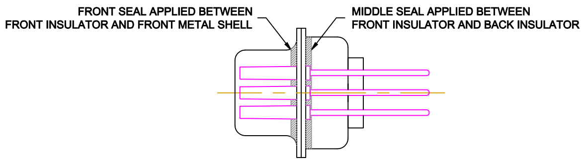
DETAIL A-A
