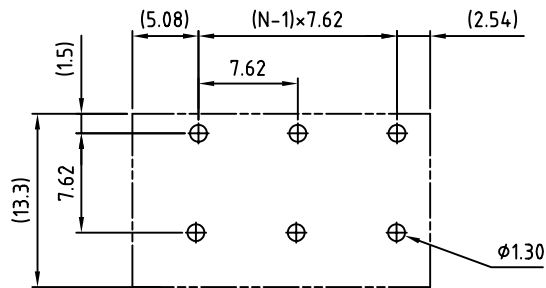
P.C.B. LAYOUT
