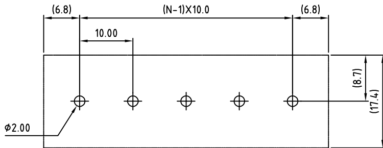
P.C.B LAYOUT
