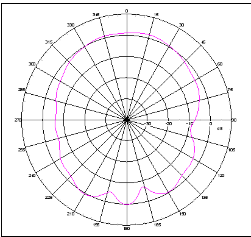
YZ-plane Free Space @1602MHz
