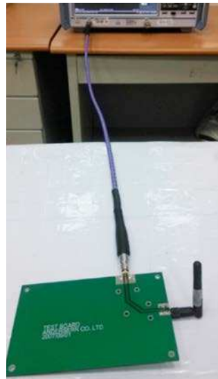
Antenna R/A
