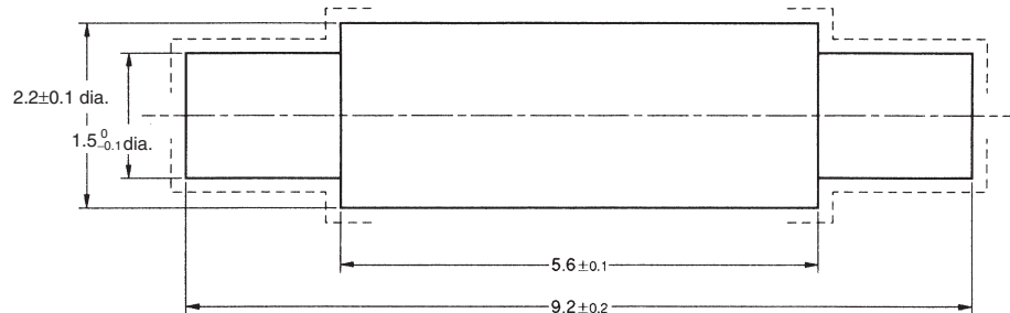
Actuator Dimensions
