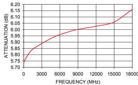
BW-S6W2+ ATTENUATION
