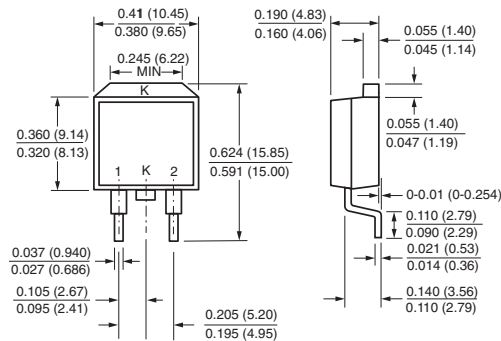
TO-263AB
