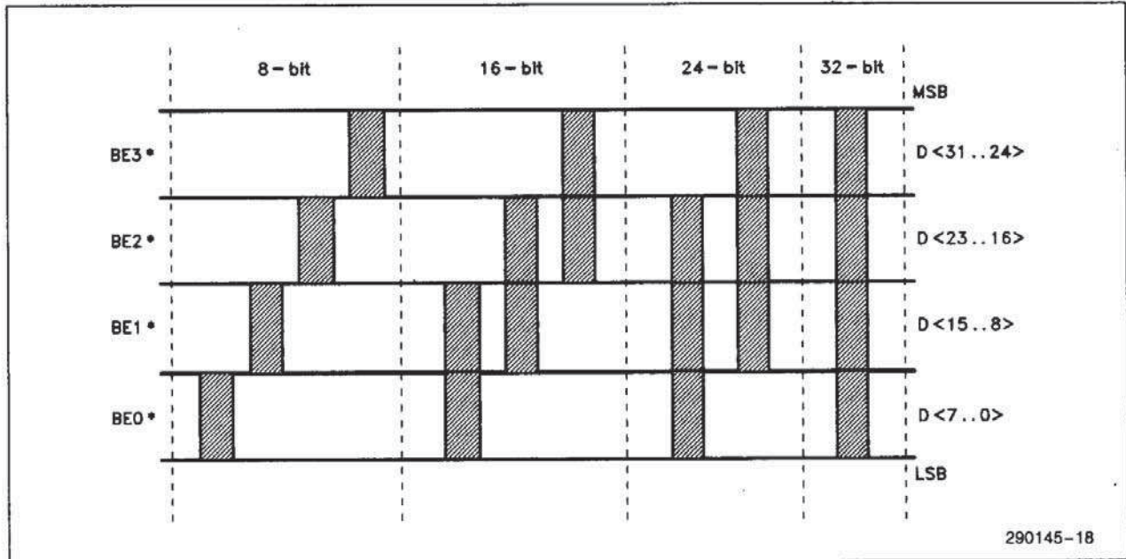
Figure 5-4. Byte Lanes
