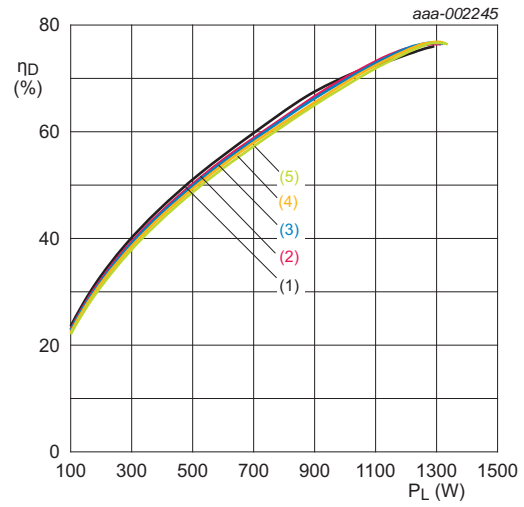
V_{DS} = 50 \text{ V}; f = 108 \text{ MHz}; t_p = 100 \text{ }\mu\text{s}; \delta = 20 \text{ \%}. (1) I_{Dq} = 0 \text{ mA} (2) I_{Dq} = 20 \text{ mA} (3) I_{Dq} = 40 \text{ mA} (4) I_{Dq} = 80 \text{ mA} (5) I_{Dq} = 160 \text{ mA}
