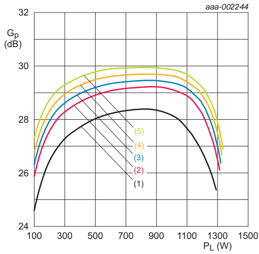
V_{DS} = 50 \text{ V}; f = 108 \text{ MHz}; t_p = 100 \text{ }\mu\text{s}; \delta = 20 \text{ \%}. (1) I_{Dq} = 0 \text{ mA} (2) I_{Dq} = 20 \text{ mA} (3) I_{Dq} = 40 \text{ mA} (4) I_{Dq} = 80 \text{ mA} (5) I_{Dq} = 160 \text{ mA}
