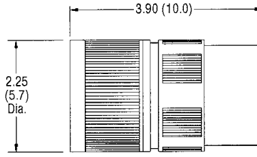
50A Connector*
