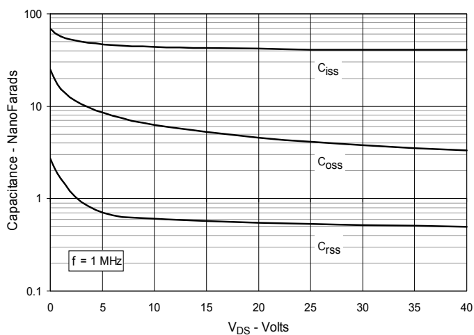
Fig. 10. Capacitance
