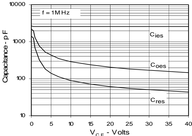
Fig. 12. Capacitance
