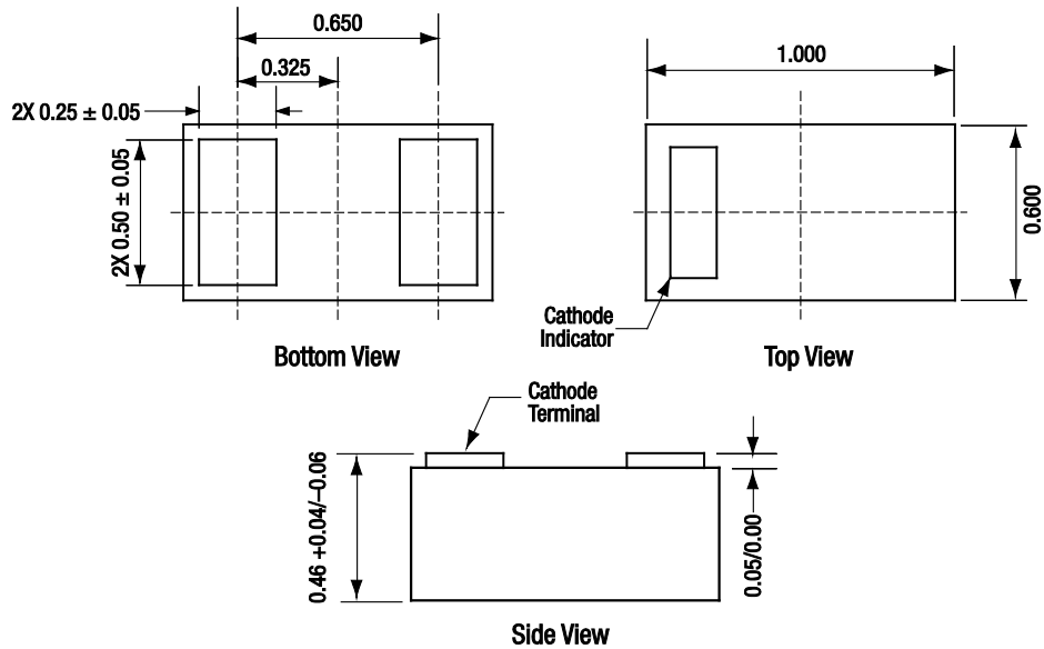
Figure 6. SMV2019-040LF Package Dimensions
