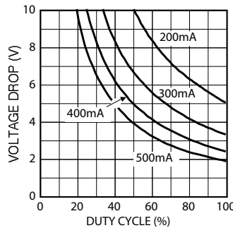
b. 50°C Ambient
