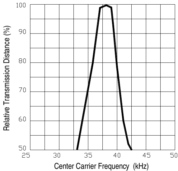
IRM-H238T/TR2
