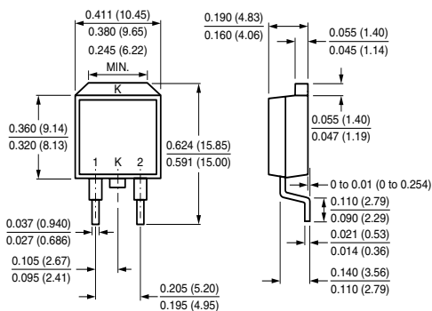
TO-263AB
