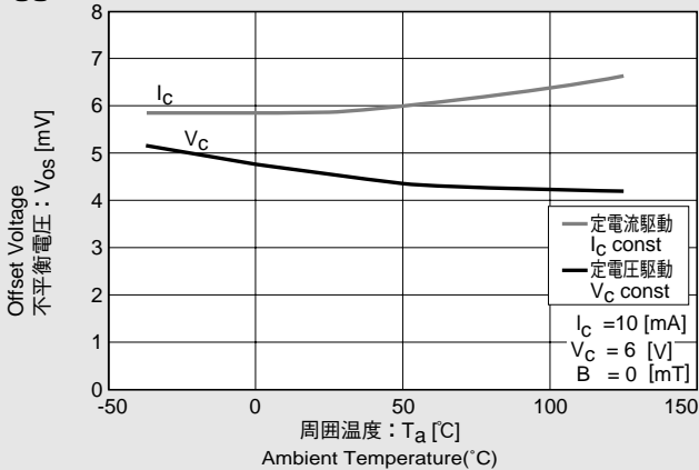
V_{OS}(V_u)-T (参考)
