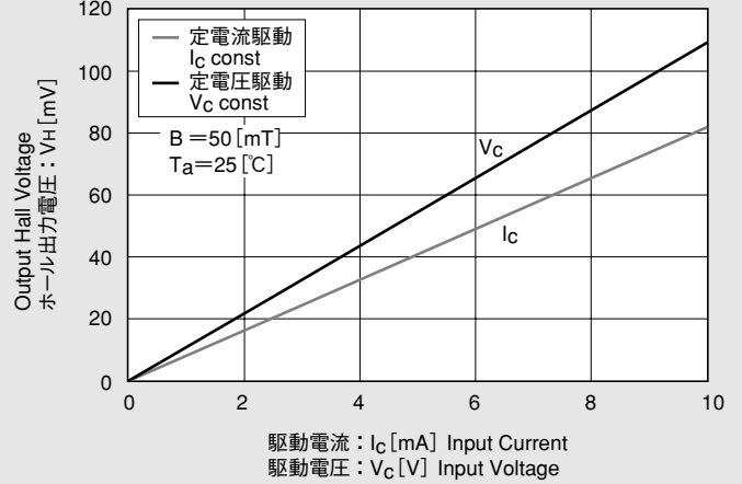
V_H-V_C, V_H-I_C
