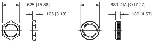
HEX NUT
