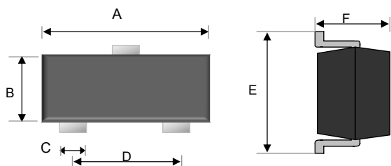
SOT-523
